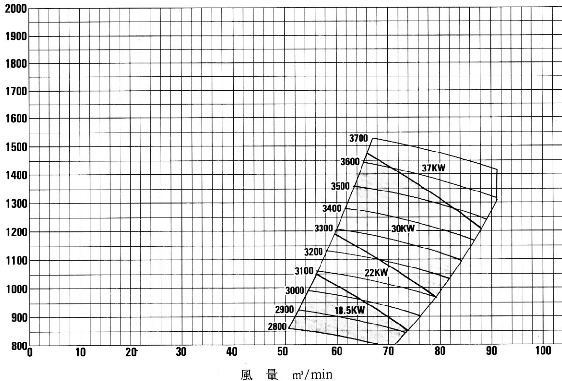
NO.5TB-2-H ターボブロアー選定図表
