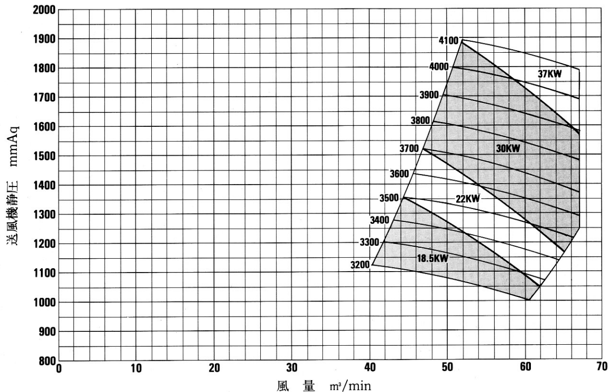
NO.5TB-1-H ターボブローワー選定図表
