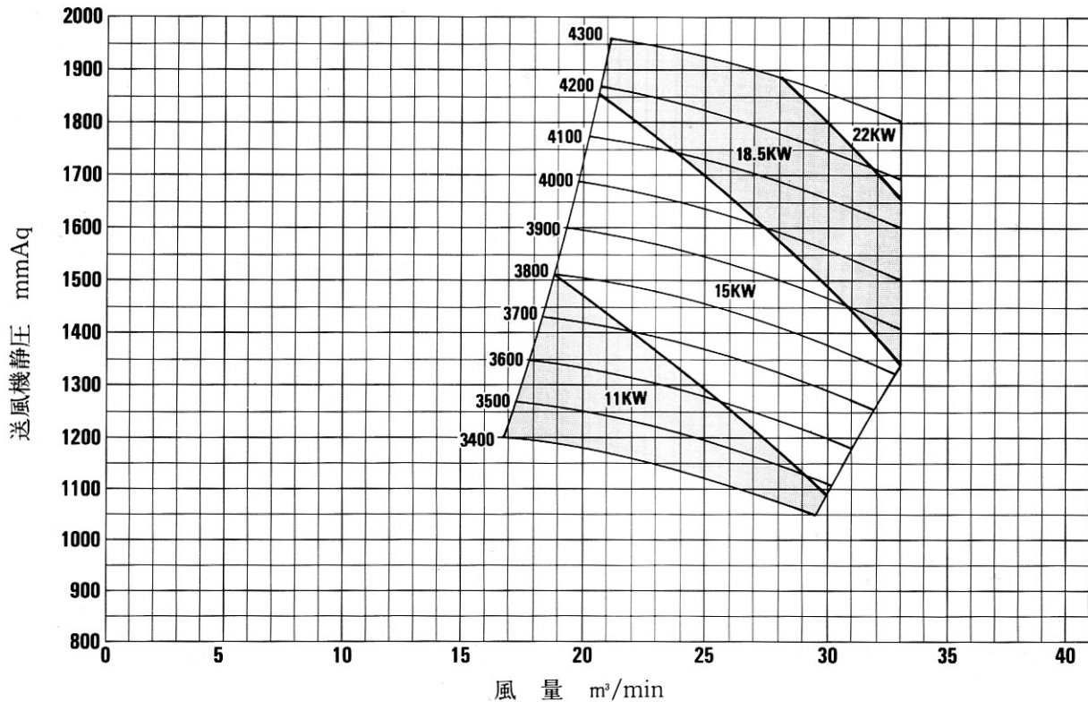
NO.4 \frac{3}{4} TB-1-H ターボブローワー選定図表
