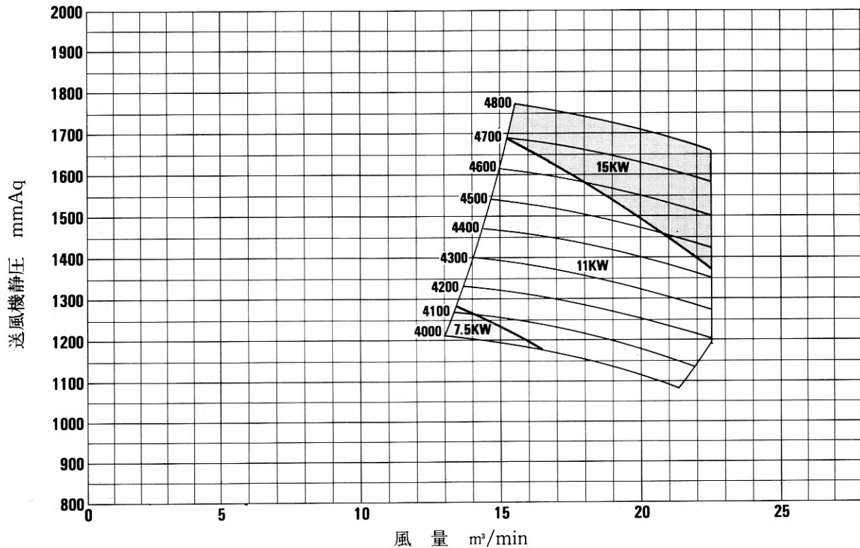
NO.4 \frac{1}{4} TB-1-H ターボブローワー選定図表
