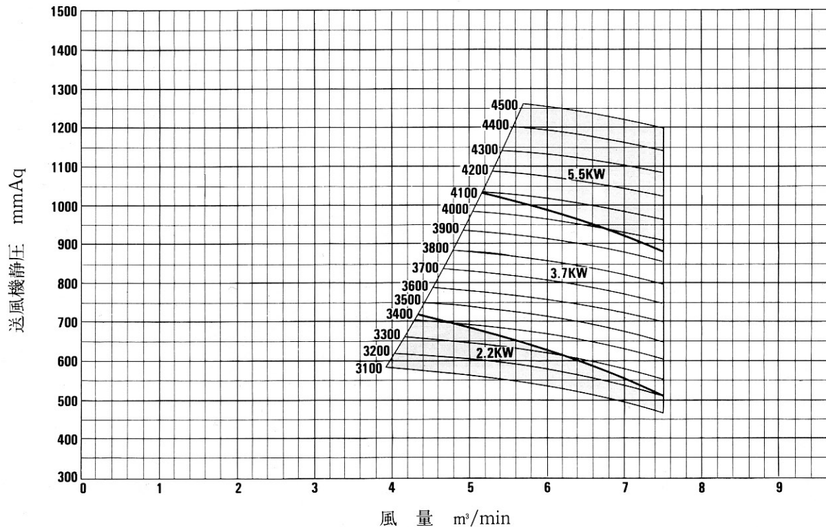
NO.4TB-1 ターボブローワー選定図表
