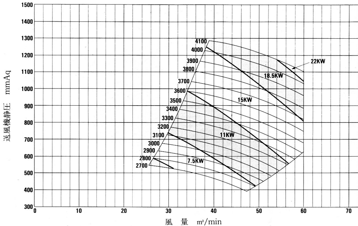
NO.4 \frac{1}{4} TB-1 ターボブローワー選定図表
