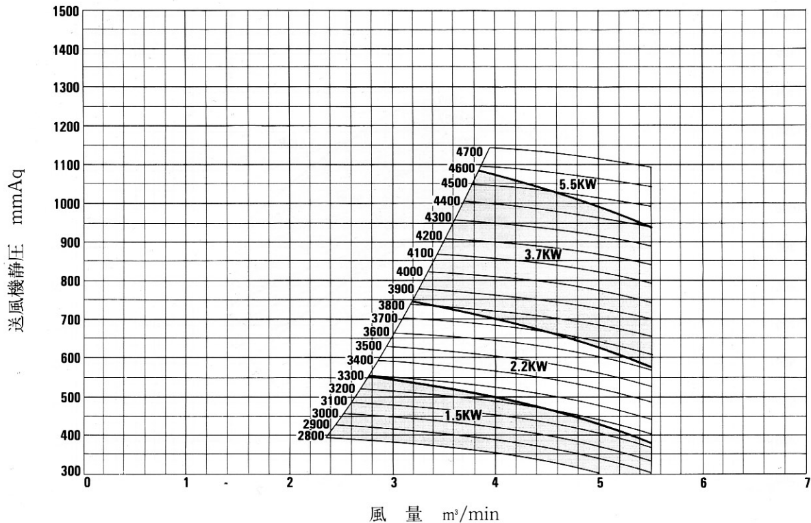
NO.3 \frac{1}{2} TB ターボブローワー選定図表
