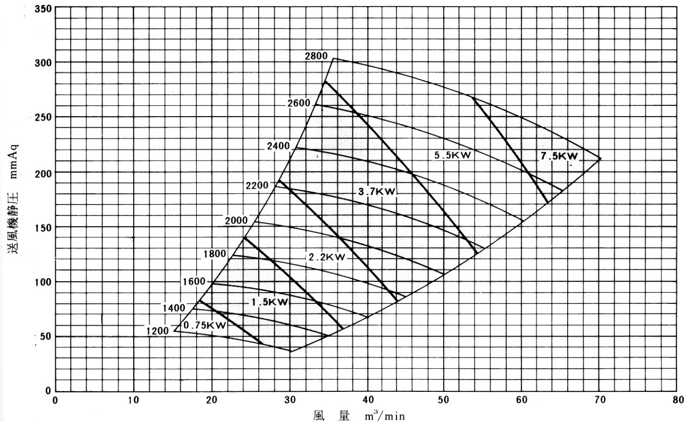
No.2 ½ プレートファン選定図表
