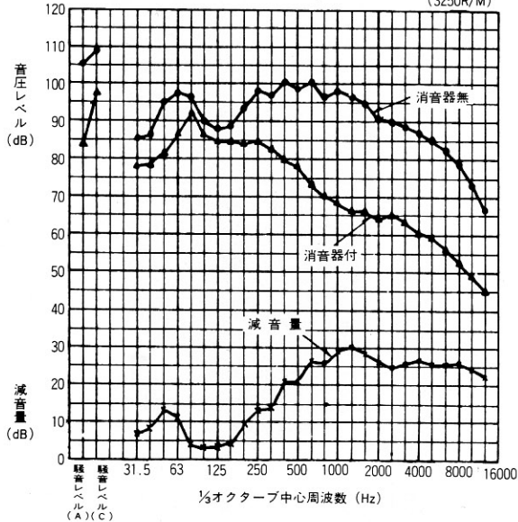
No. 3 ターボファン周波数分析
