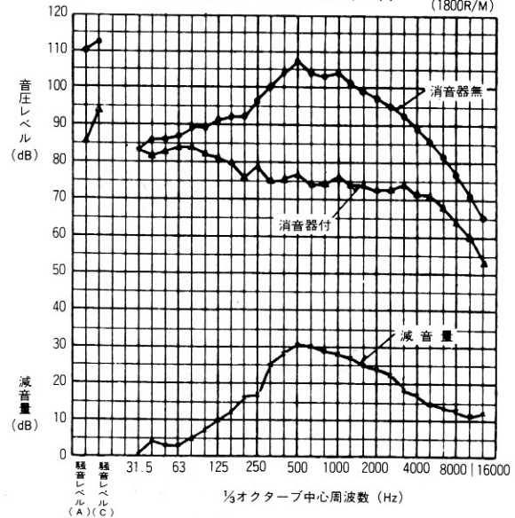
φ 800軸流ファン周波数分析
