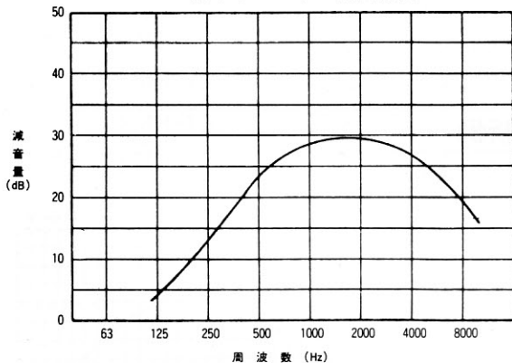
MH型サイレンサー減衰特性
