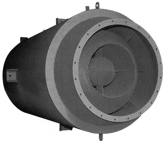
2000m 3 /min用サイレンサー 減音量35dB(A)
