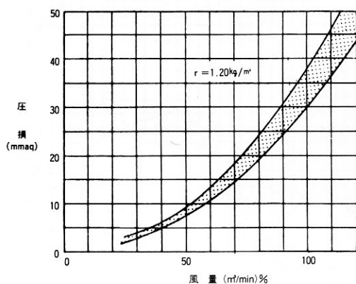
MH形サイレンサー抵抗曲線
